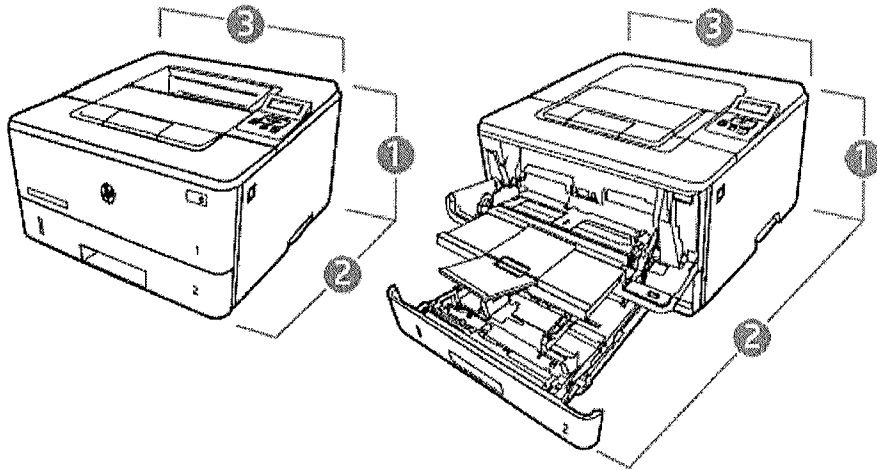
Dimensões para os modelos M304, M305, M404 e M405
